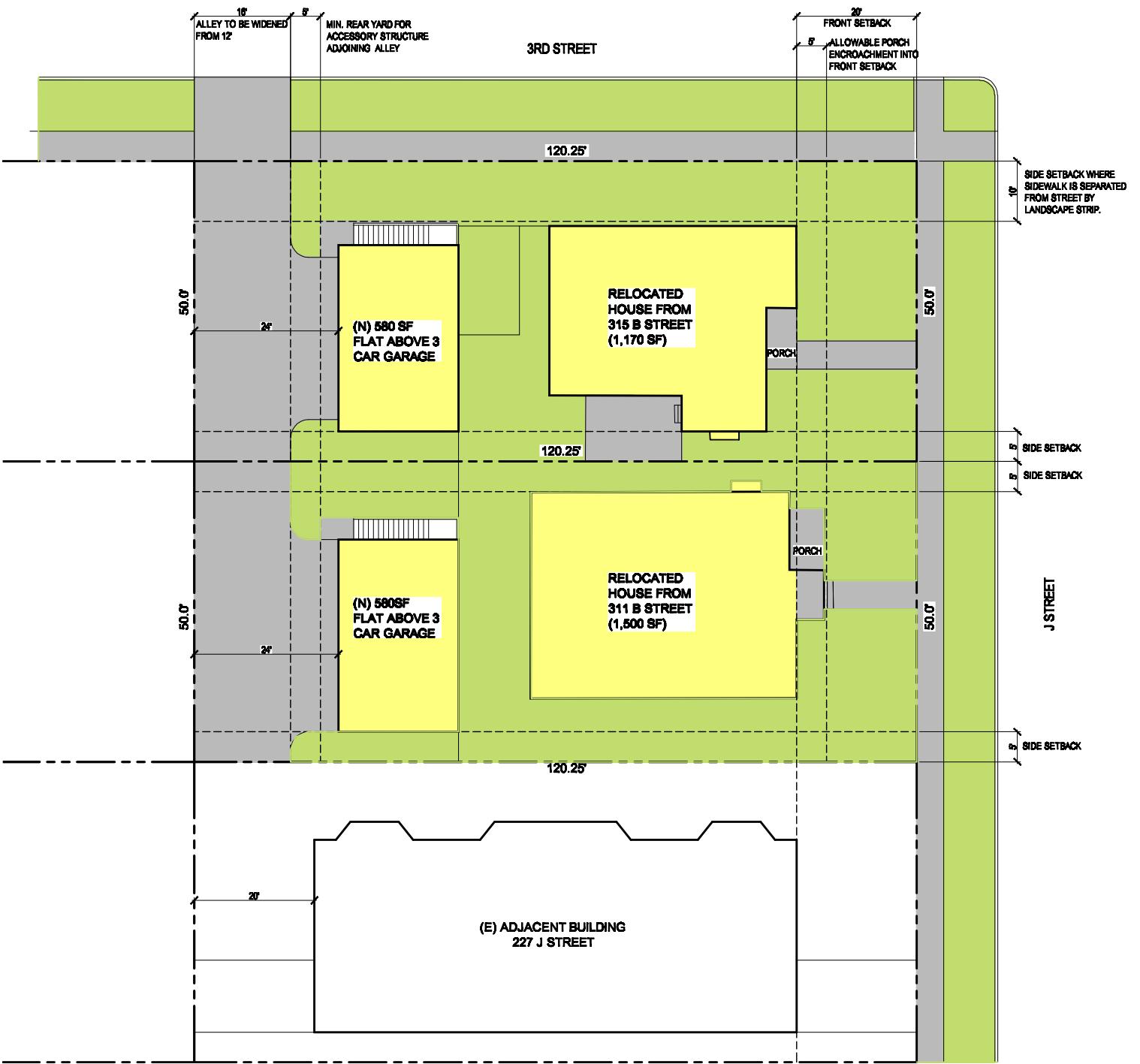
SITE PLAN - OPTION B
